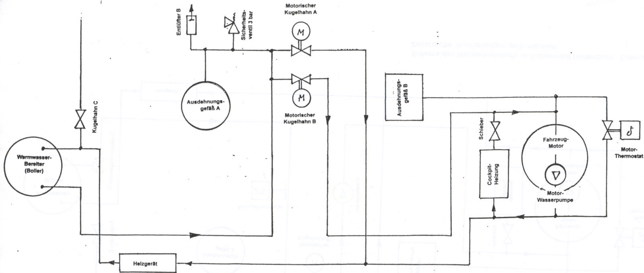
Schema des Wasserkreislaufs im Reisemobil Gertenbach Entwurf x278.3 Jetziger Ausbauzustand
